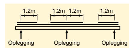
Overzicht kruisnetten
